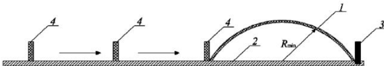
1 - образец; 2 - поверхность стенда; 3 - фиксированный упор; 4 - подвижный упор
