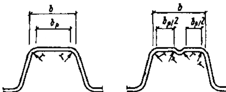
Рис. 5. К определению ширины плоских участков сжатых полок
